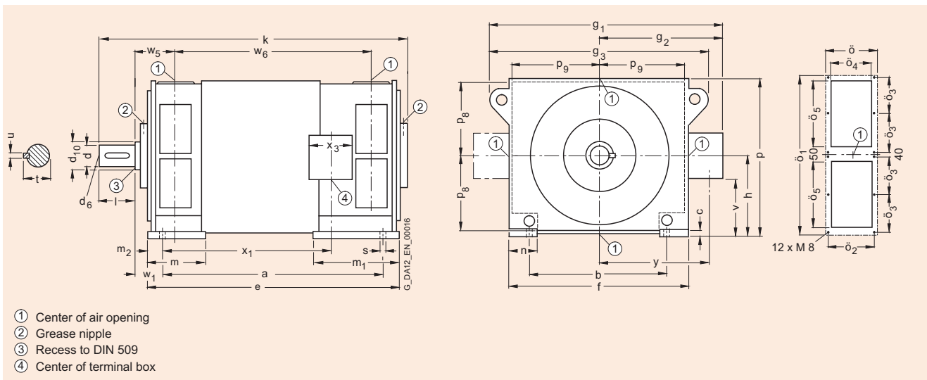
Type IM B 3
