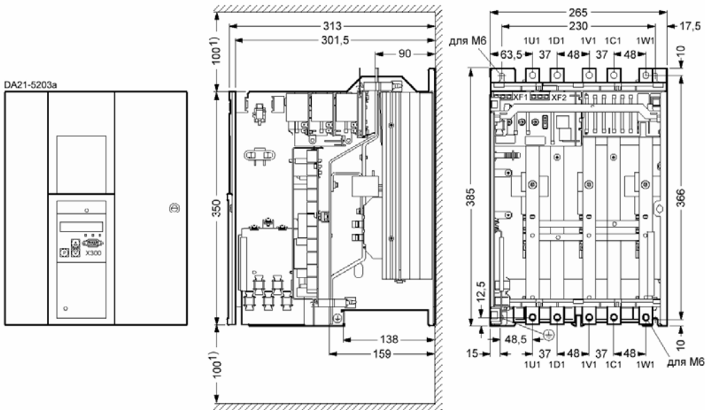
Рис. 8/14 AC 460 V, 210 A ... 280 A, 1Q
