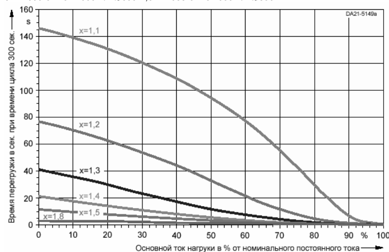
Рис. 5/21 6RA7090-6GV62 1100 A/4Q/575 V Siemens DA21.1 · 2001
