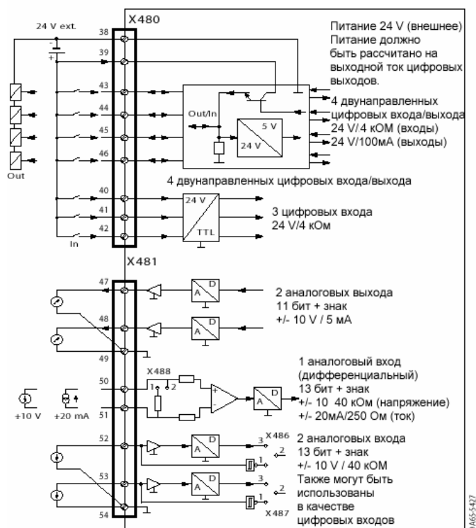
Рис. 4/11 Схема модуля расширения клемм EB1
