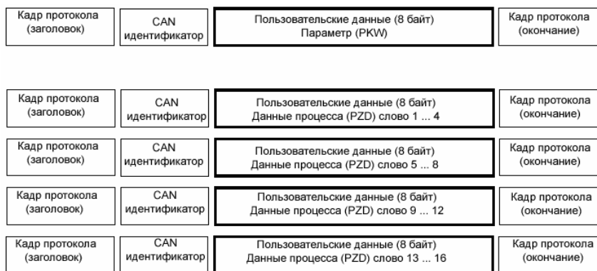
Рис. 4/28 Структура пользовательских данных в телеграмме.
