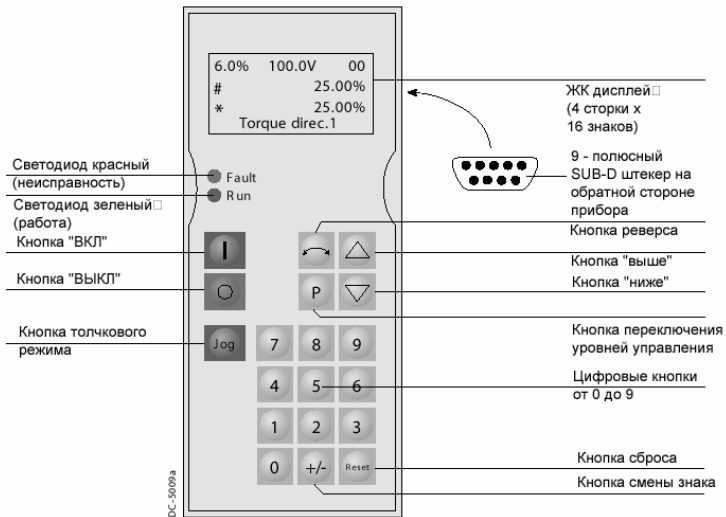
Рис. 4/31 Внешний вид OP1S
