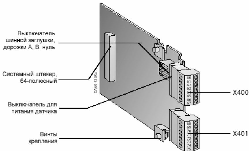
Рис. 4/9 Оptionальный модуль SPB
