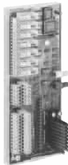
Рис. 4/15 Интерфейсный модуль SCI2
