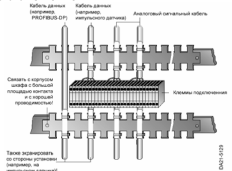
Рис. 5/37 Экранирование в электрическом шкафу.
