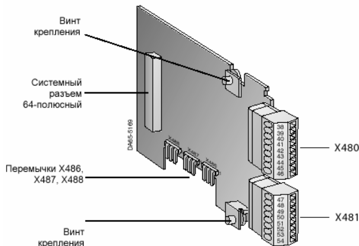
Рис. 4/10 Модуль расширения клемм EB1
