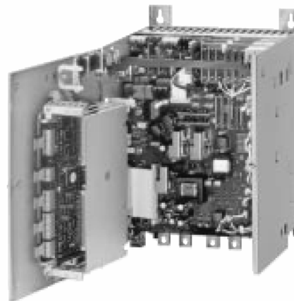
Рис. 2/2 SIMOREG 6RA70, 15А/30А
