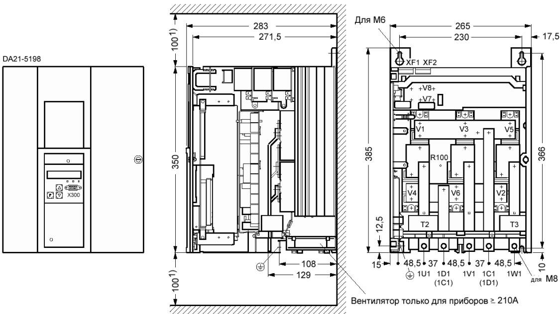
Рис. 8/9 1) Следует обеспечить минимальное пространство для циркуляции воздуха, для подвода достаточного количества воздуха
