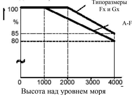
Рис.2-3. Влияние высоты установки привода
