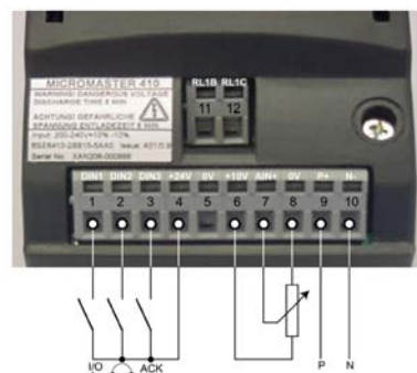
Блок-схема преобразователя MICROMASTER 410
