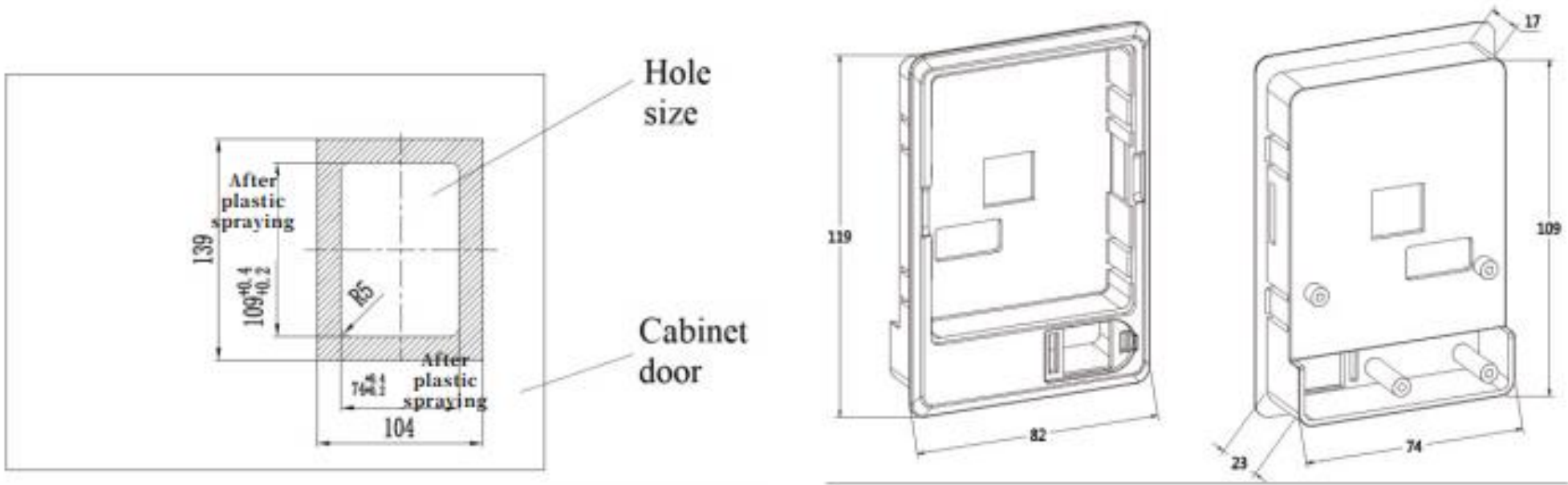
Схема отверстий на двери шкафа для монтажа простой клавиатуры
